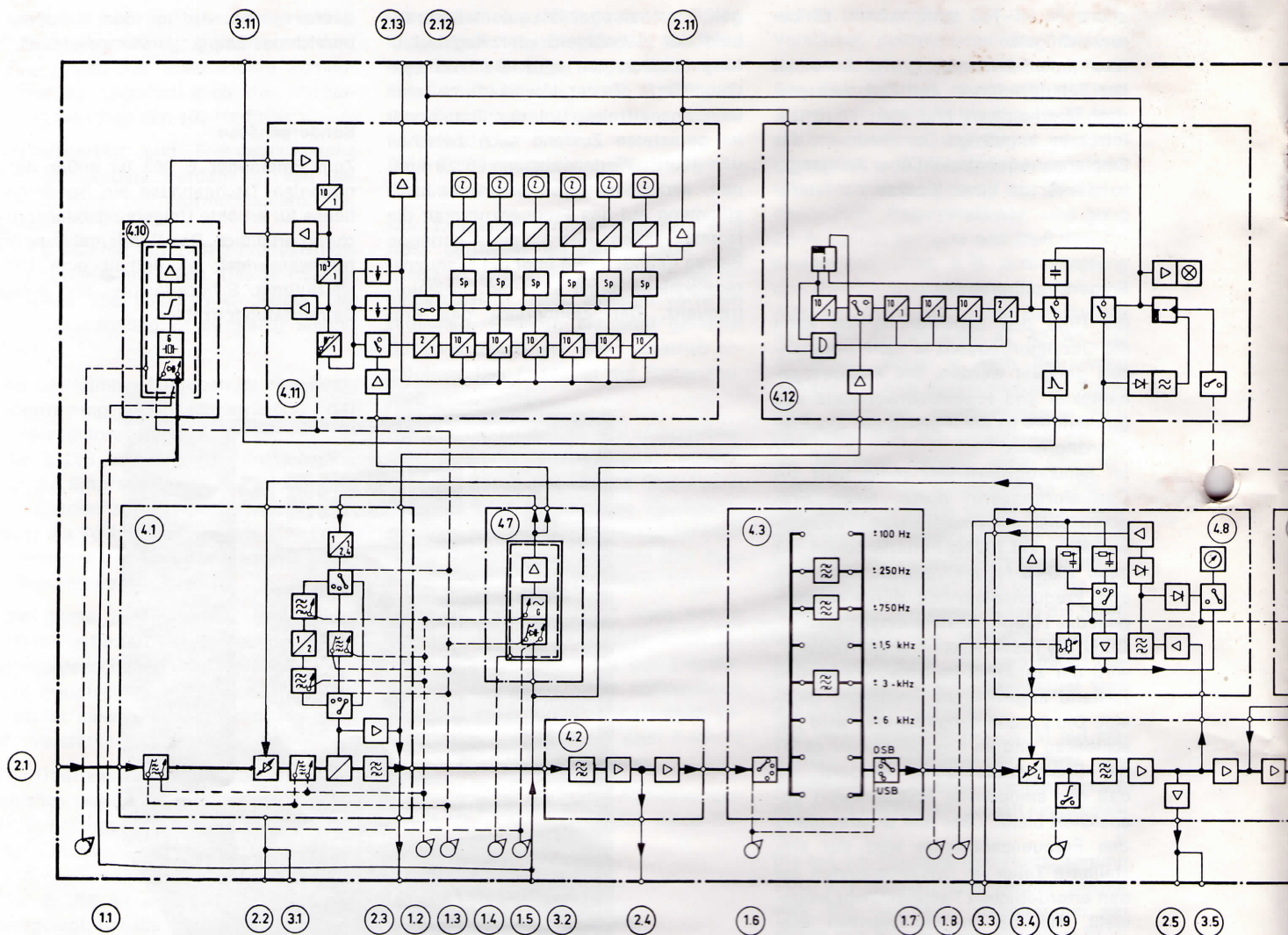
Blockschaltbild des KW-Empfängers E 863 KW/2
